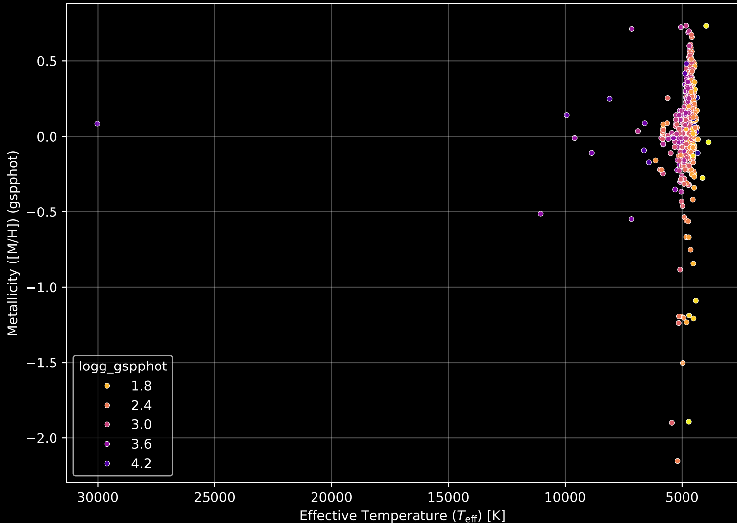
APOGEE DR17 Field: [335+06] Stellar Population Parameters (n= 587)
